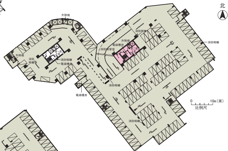
平台四樓平面圖
