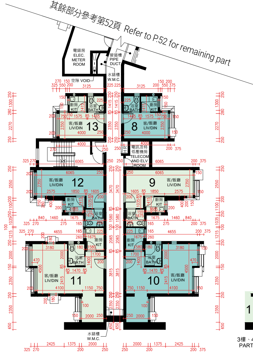
4樓、13樓及22樓部分平面圖 PART PLAN OF 4/F, 13/F & 22/F
