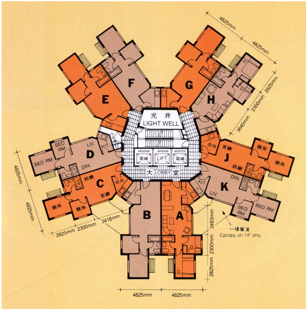
樓宇樣本平面圖 海福花園第1座
