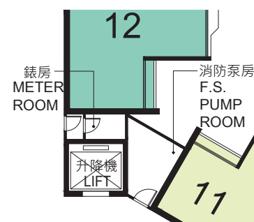
18樓部分平面圖 PART PLAN OF 18/F
