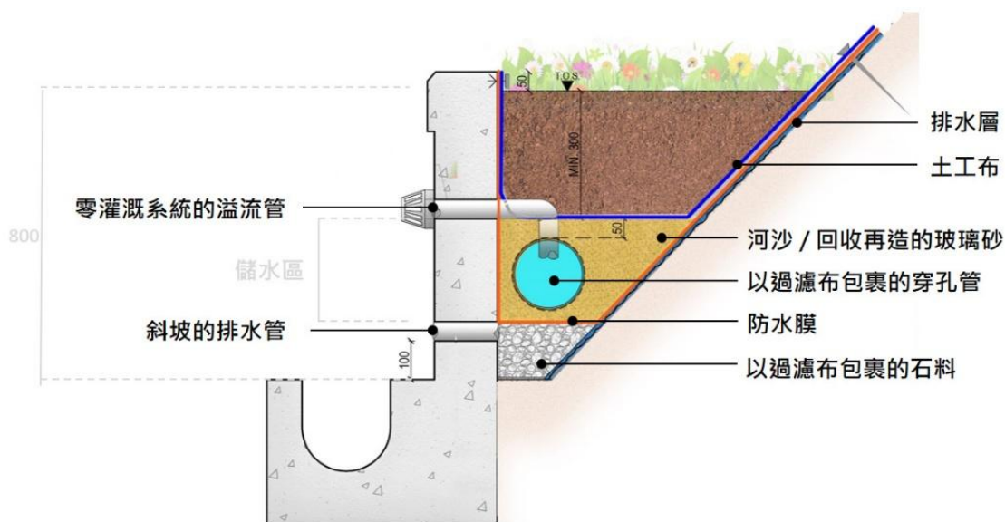
魷魚灣村路的零灌溉系統（加強版）設計。
