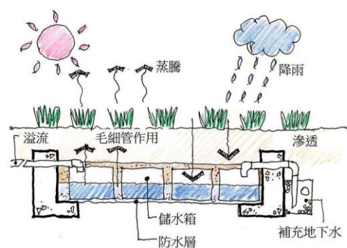
零灌溉系統的設計理念。
